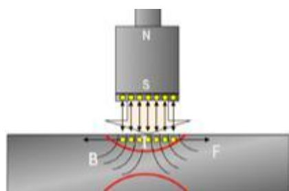
Принцип работы ЭМА преобразования
